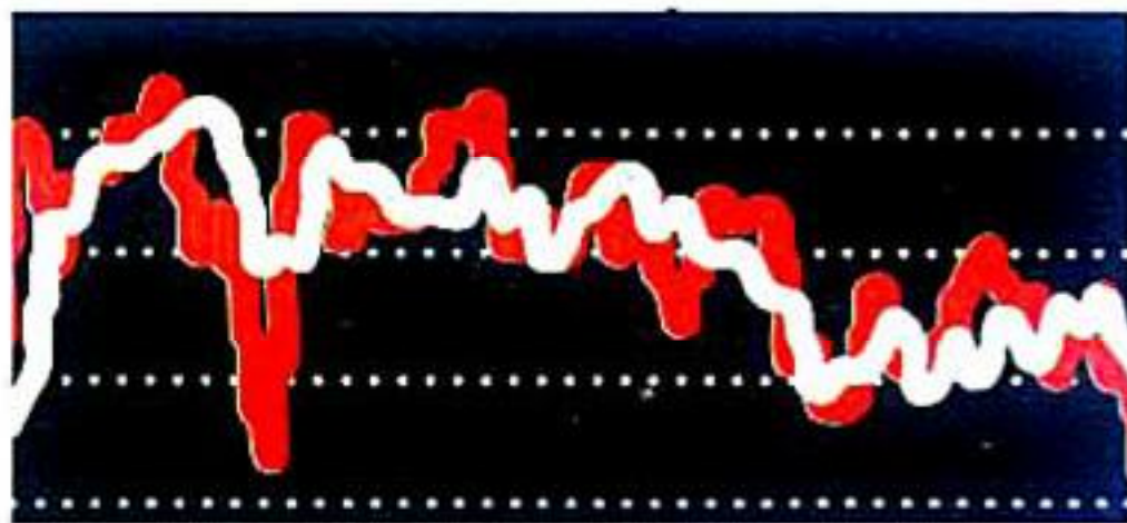
Das 'AR Acoustic Blanket' glättet den Frequenzgang der Mittel- und Hochtönsysteme. Die rote Kurve zeigt den Frequenzgang der AR91 von ca. 6000 bis 18000 Hz ohne akustische Bedämpfung durch das Acoustic Blanket. Die weiße Kurve stellt den gradlinigeren Frequenzgang bei derselben Anlage mit Acoustic Blanket dar.
